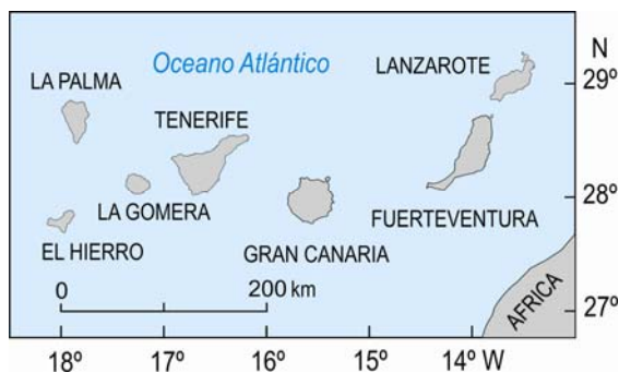
Fig. 1: Situación geográfica de las Islas Canarias. En las Canarias Orientales se han hallado los principales testimonios paleoclimáticos.
